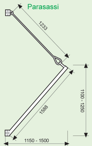
Mensola per sbalzo
